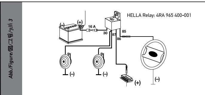
รูปที่ 3: วิธีการเดินสายไฟที่เหมาะสมสำหรับแตรรูปจานของ HELLA
